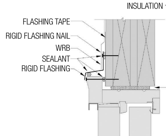
FIG. 18: HEAD JAMB
