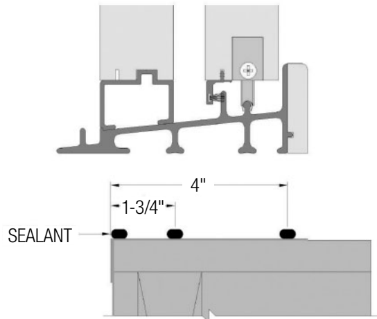
FIG. 11: SLIDING PATIO DOOR SILL
