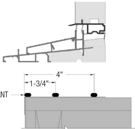
FIG. 10: 4-9/16" & 6-9/16" IN-SWING PATIO DOOR SILL
