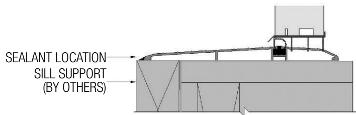
FIG. 16: HANDICAP DOOR SILL
