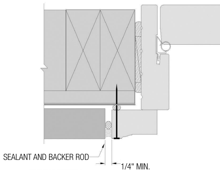
FIG. 20: SIDE JAMB
