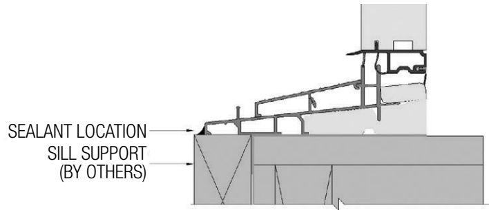
FIG. 15: STANDARD DOOR SILL
