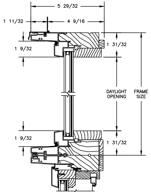
TRANSOM HEAD JAMB & SILL
