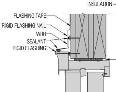
FIG. 17: HEAD JAMB
