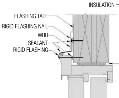
FIG. 17: HEAD JAMB
