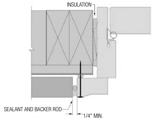
FIG. 19: SIDE JAMB
