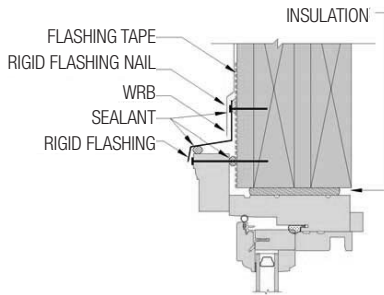
FIG. 14: HEAD JAMB
