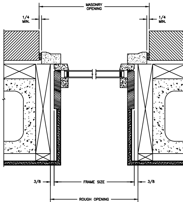
JAMBS 8\"/>
