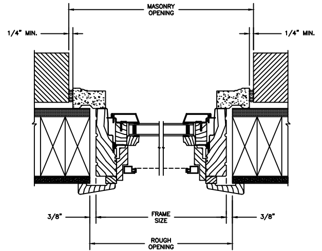
JAMB
