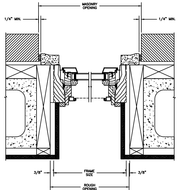
JAMB
