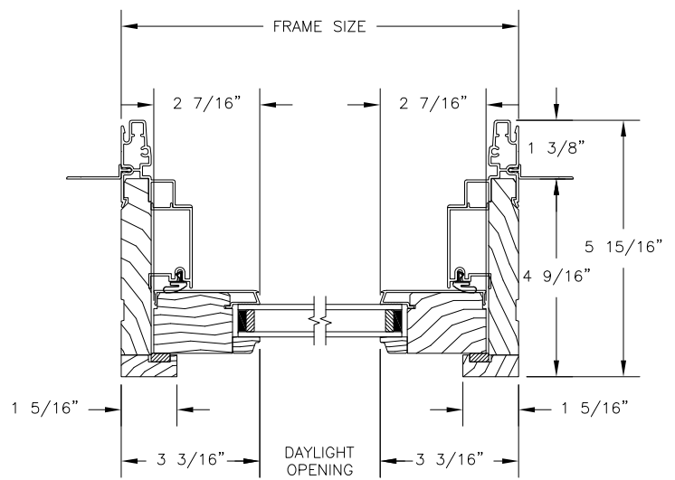
JAMBS
