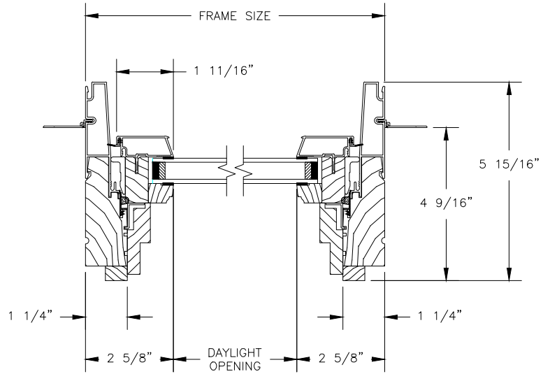
JAMBS
