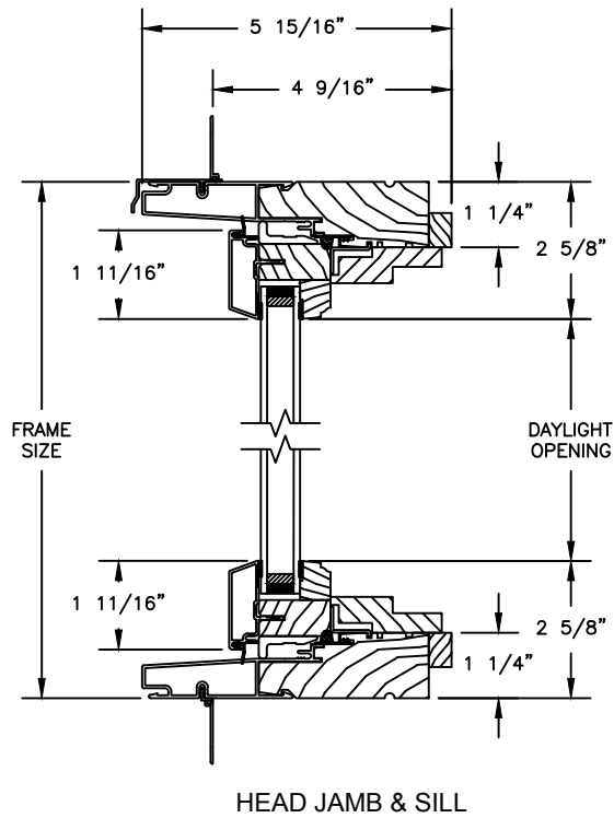
TRANSOM
