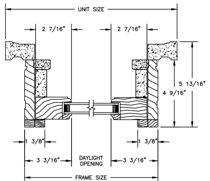
JAMBS
