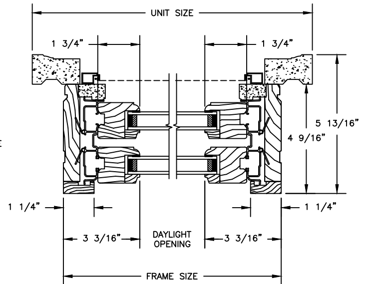
JAMBS
