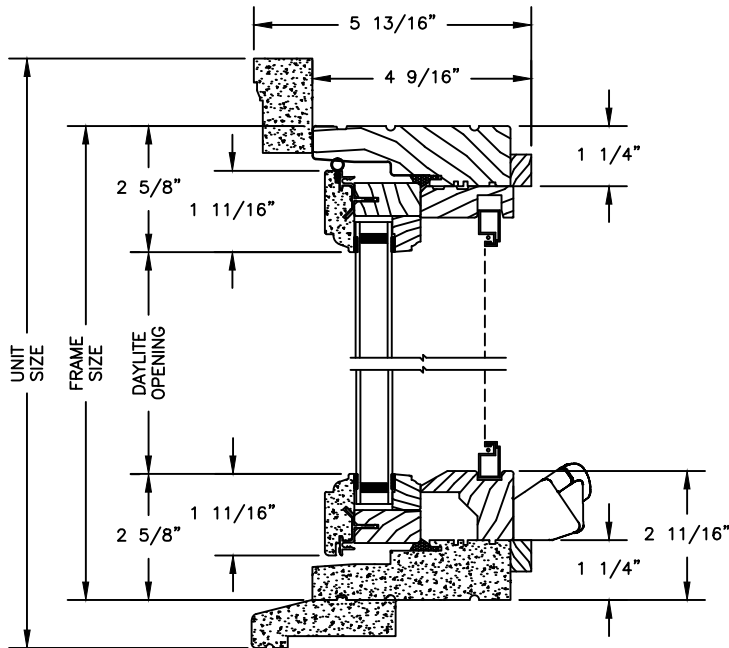
HEAD JAMB & SILL
