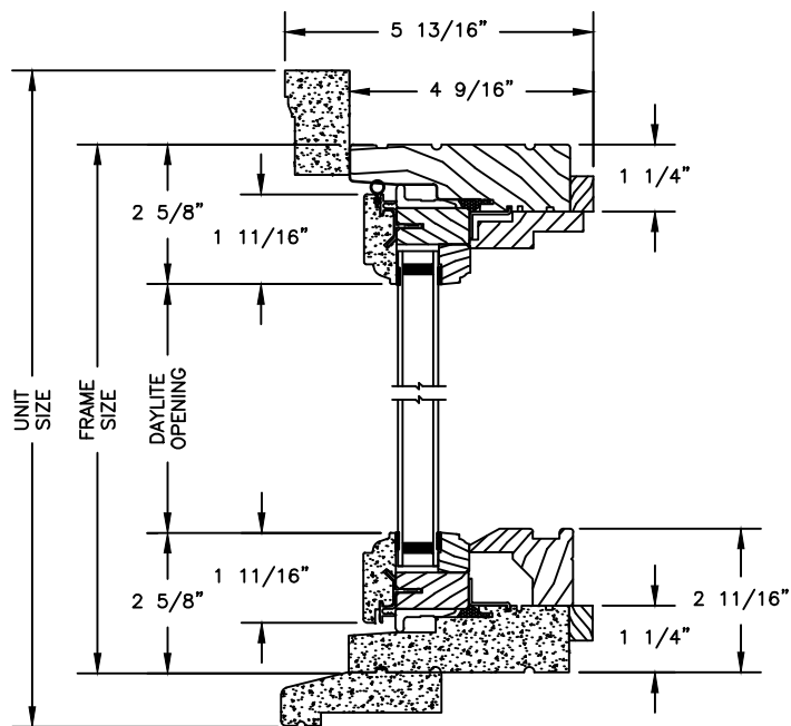
HEAD JAMB & SILL
