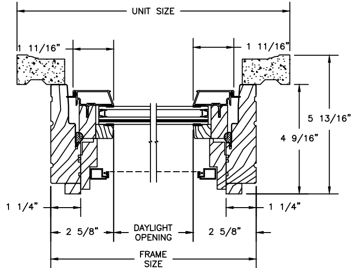
JAMBS
