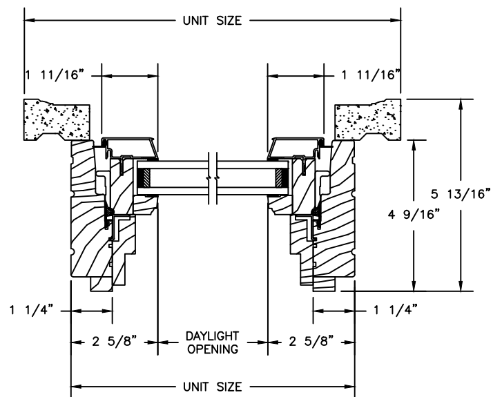
JAMBS
