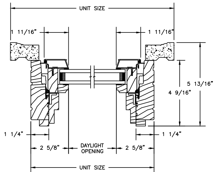
JAMBS
