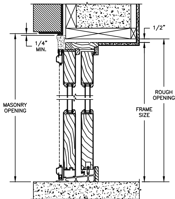
HEAD JAMB & SILL 8\"/>
